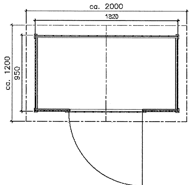
Grundriss und Fundamentplan (2 + 4 Fundamenthölzer)
