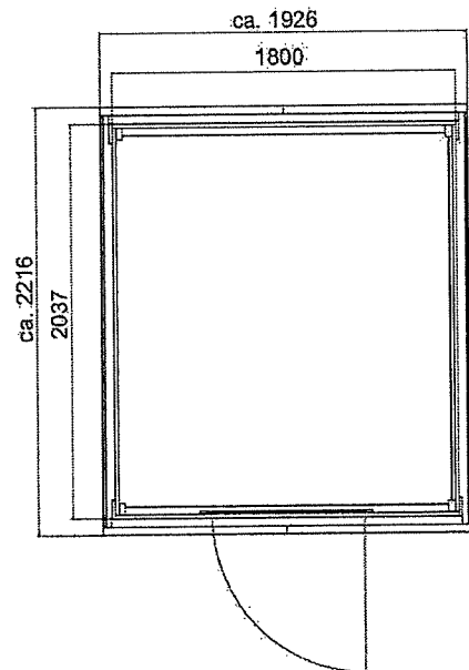
Grundriss und Fundamentplan (4 Fundamenthölzer)
